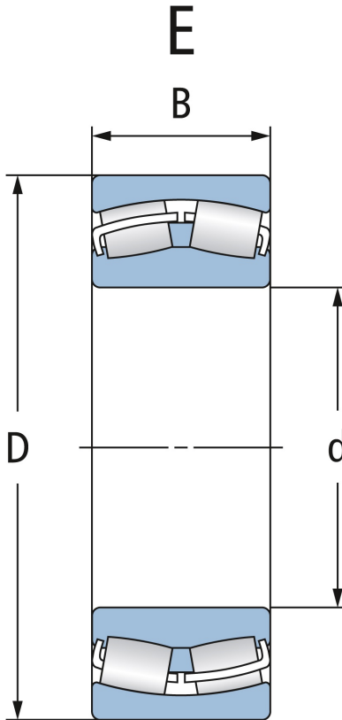
Zylindrische Bohrung Cylindrical bore
